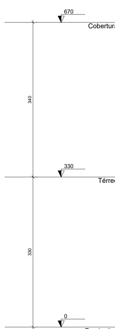
02 CORTE C-C escala 1:50
