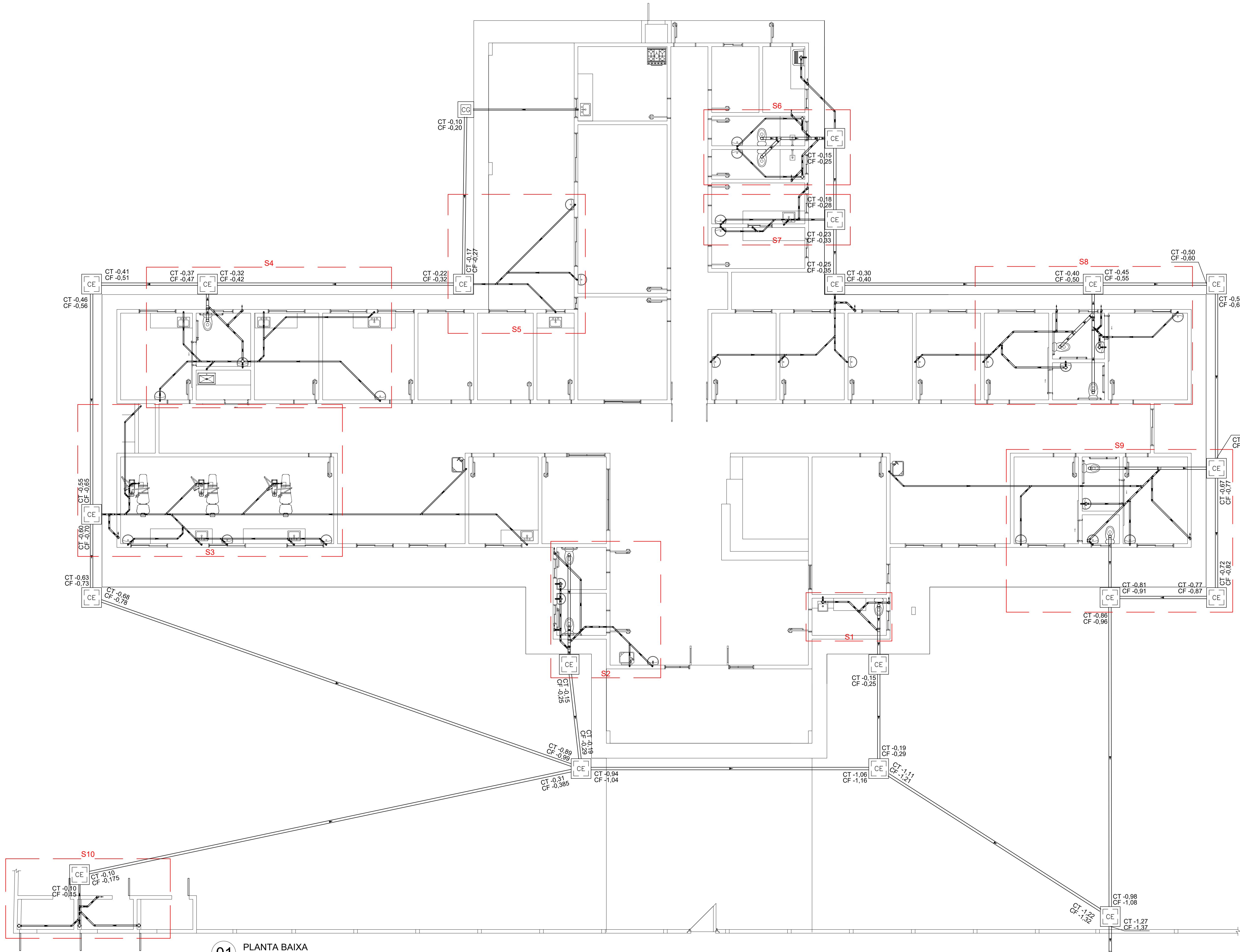
01 PLANTA BAIXA 1 : 75
