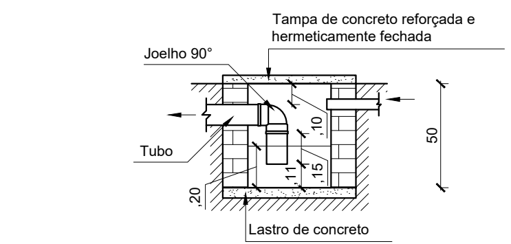
03 CAIXA DE GORDURA SIMPLES - CORTE 1 : 25
