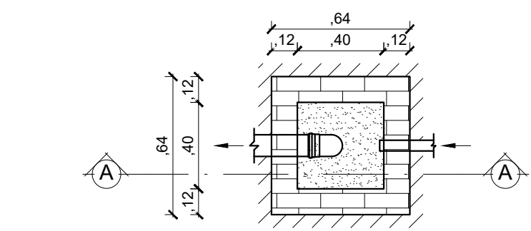
02 CAIXA DE GORDURA SIMPLES - PLANTA 1 : 25
