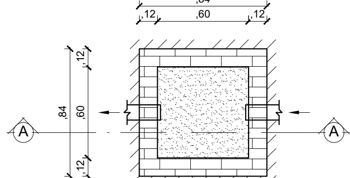
05 CAIXA DE INSPEÇÃO - PLANTA 1 : 25
