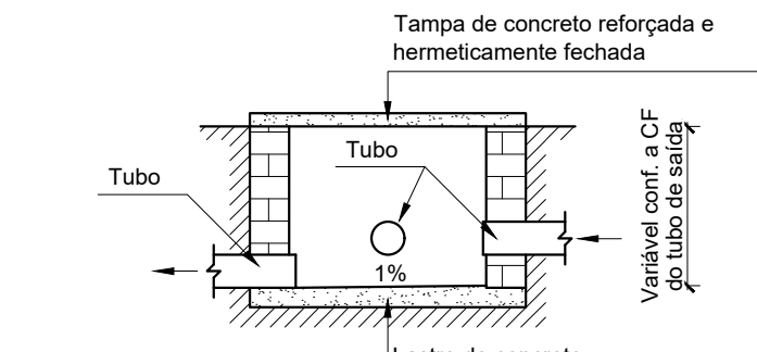
04 CAIXA DE INSPEÇÃO - CORTE 1 : 25
