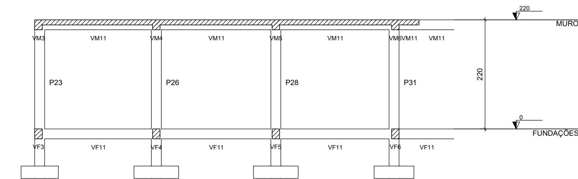
02 Corte A-A escala 1:75
