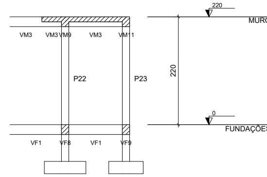
04 Corte A-A escala 1:75
